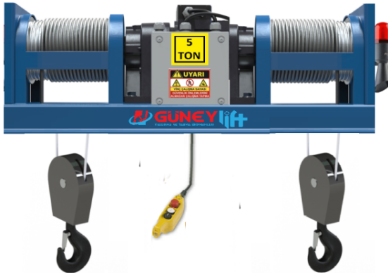
5 TON ÇİFT TAMBUR ASANSÖR VİNC SİSTEMİ
